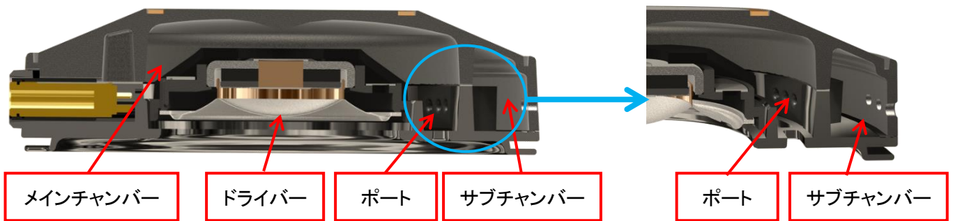
【ハウジング断面図】
